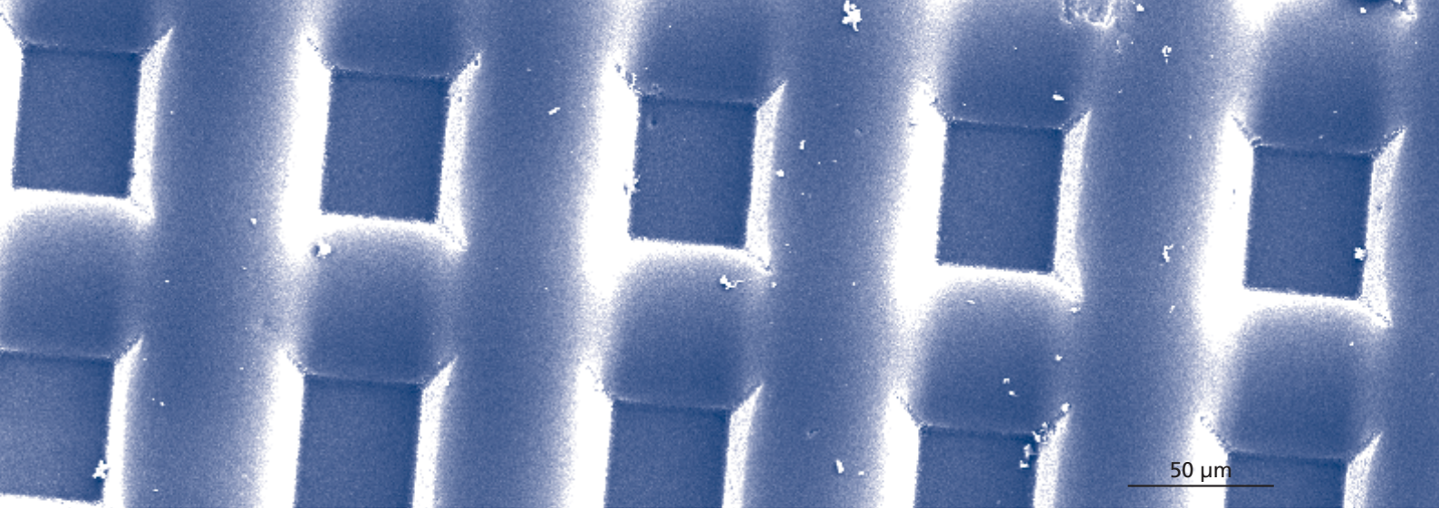
Mikrometerfeine strukturierte Polystyroloberfläche für mikrofluidische Anwendungen.
